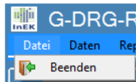
Abb. 12: Menüpunkt "Datei"
