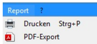
Abb. 15: Menüpunkt "Report"
